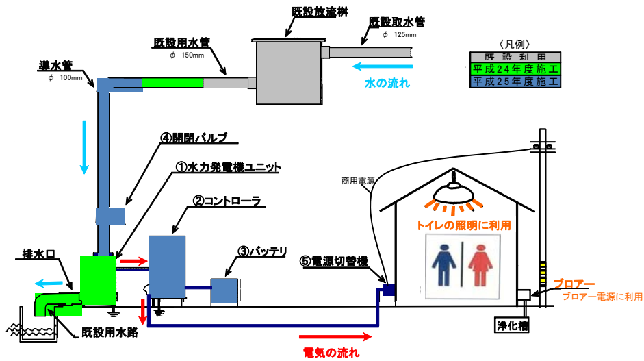
四谷 小水力発電施設 全体構成図
